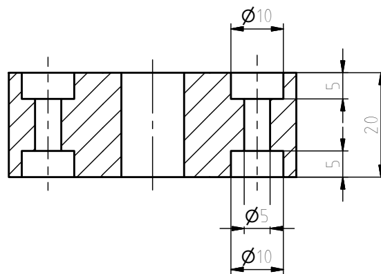
A-A (1:1)
