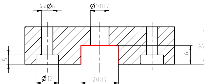
A-A (1:1)
