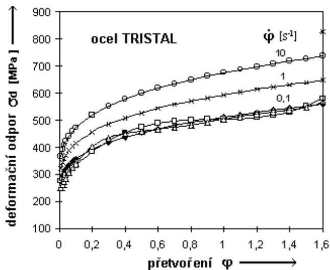
Obr.1 Křivky napětí-deformace
